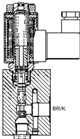
Schnitt B-B
